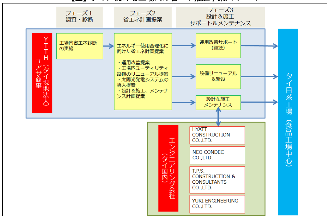
【図】タイにおける工場向け省エネ推進事業スキーム
